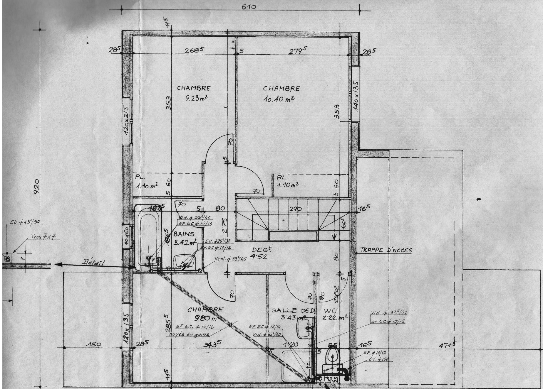
Poterne (type CB) : plan plomberie - étage (original de 1980)
