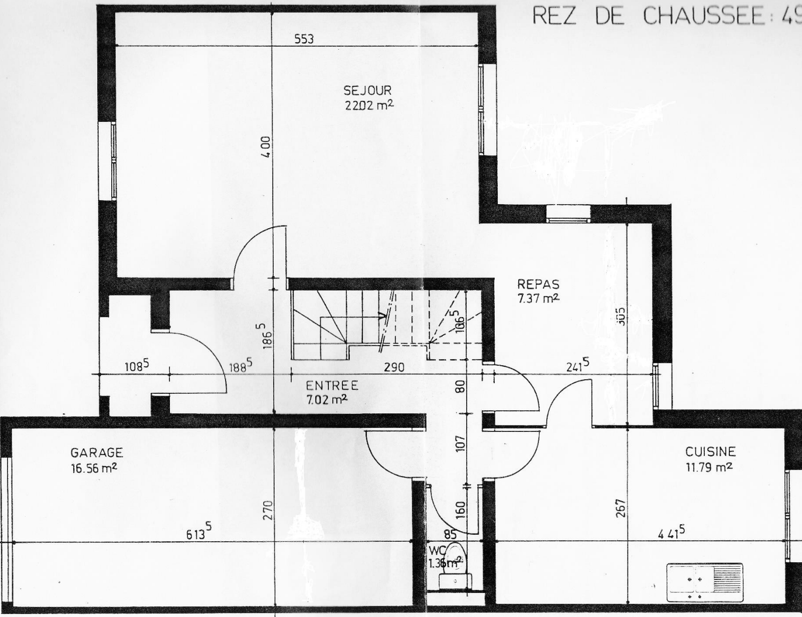
Poterne (type CB) : plan général (original de 1980)
