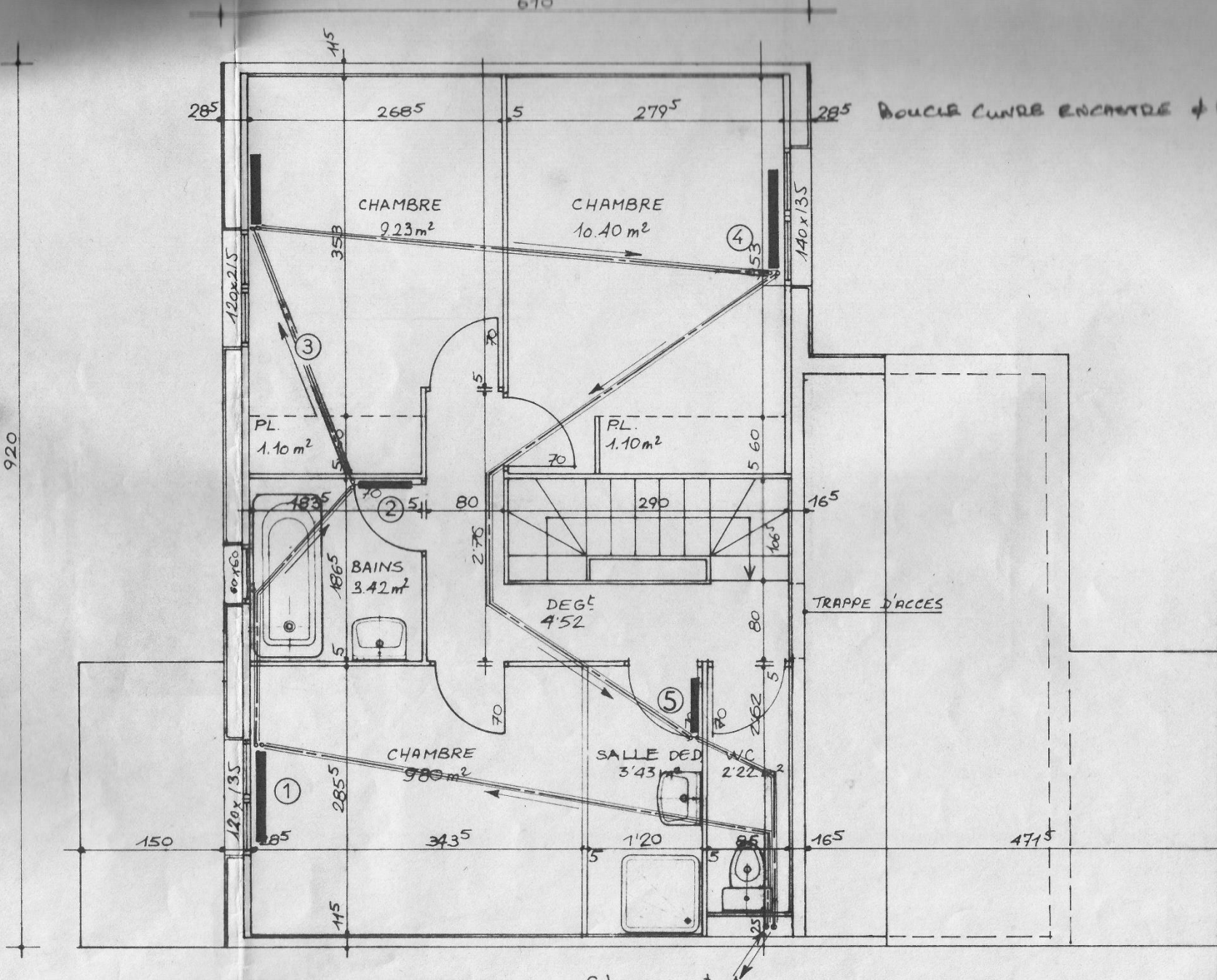
Poterne (type CB) : plan chauffage - étage (original de 1980)
