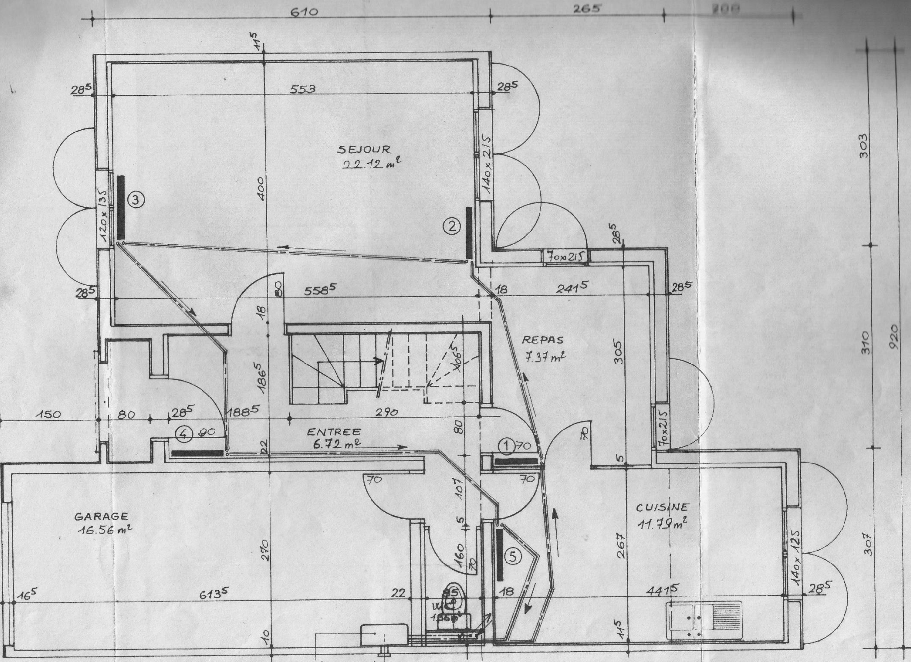
Poterne (type CB) : plan chauffage – rez-de-chaussée (original de 1980)
