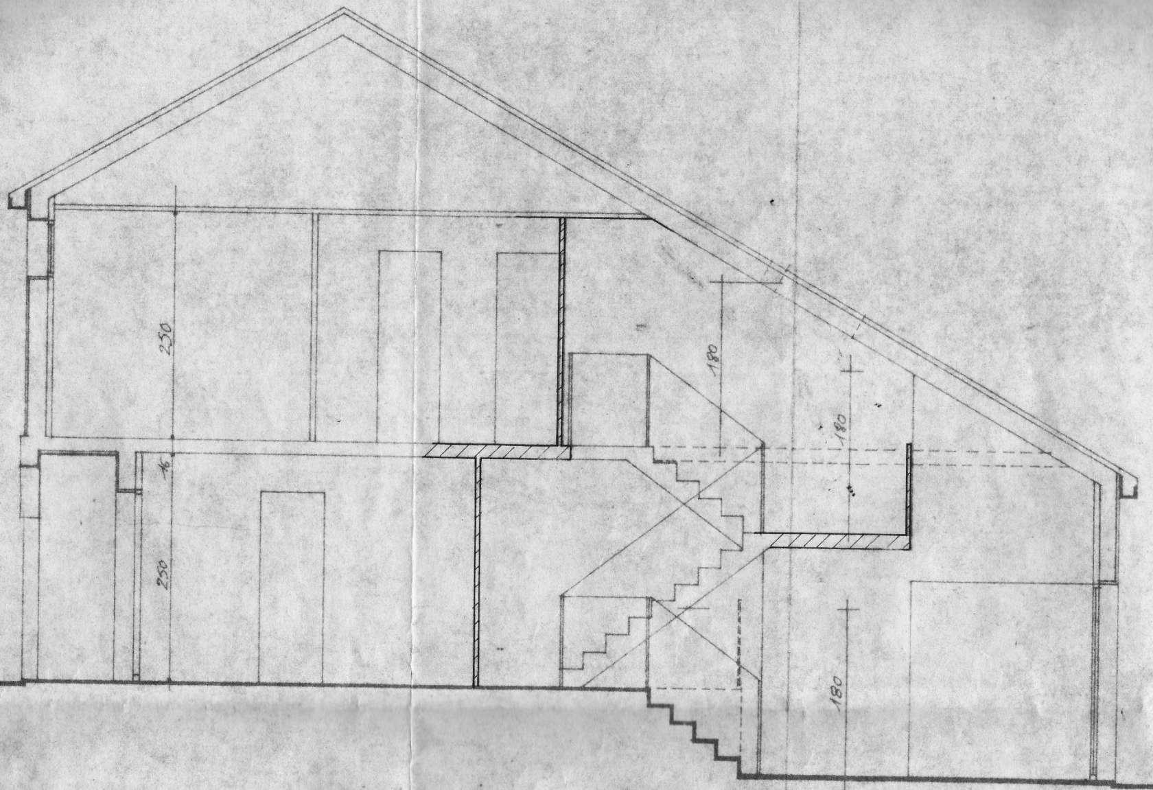
Echaugette (type B1) : plan de coupe (original de 1980)
