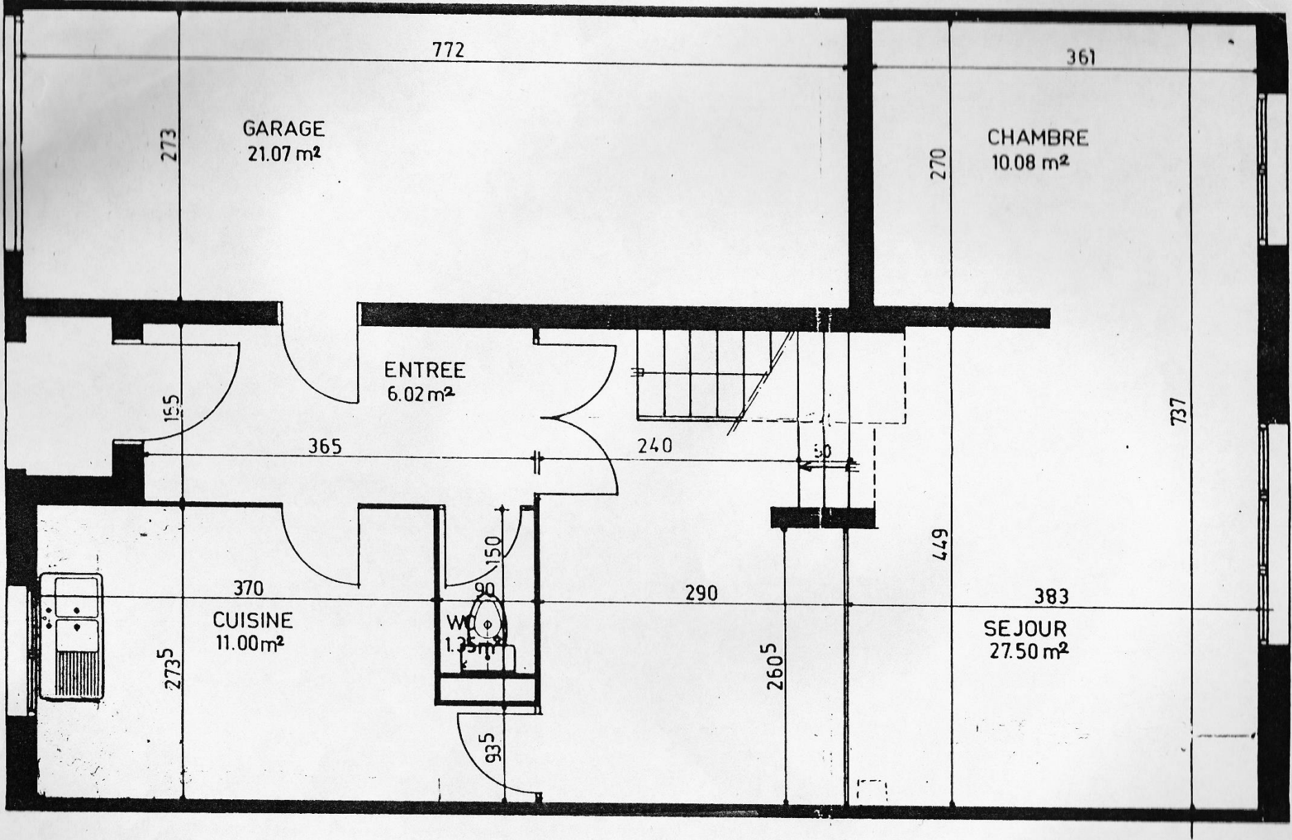
Echaugette (type B1) : plan général - rez-de-chaussée → 55,95 m 2 (original de 1980)
