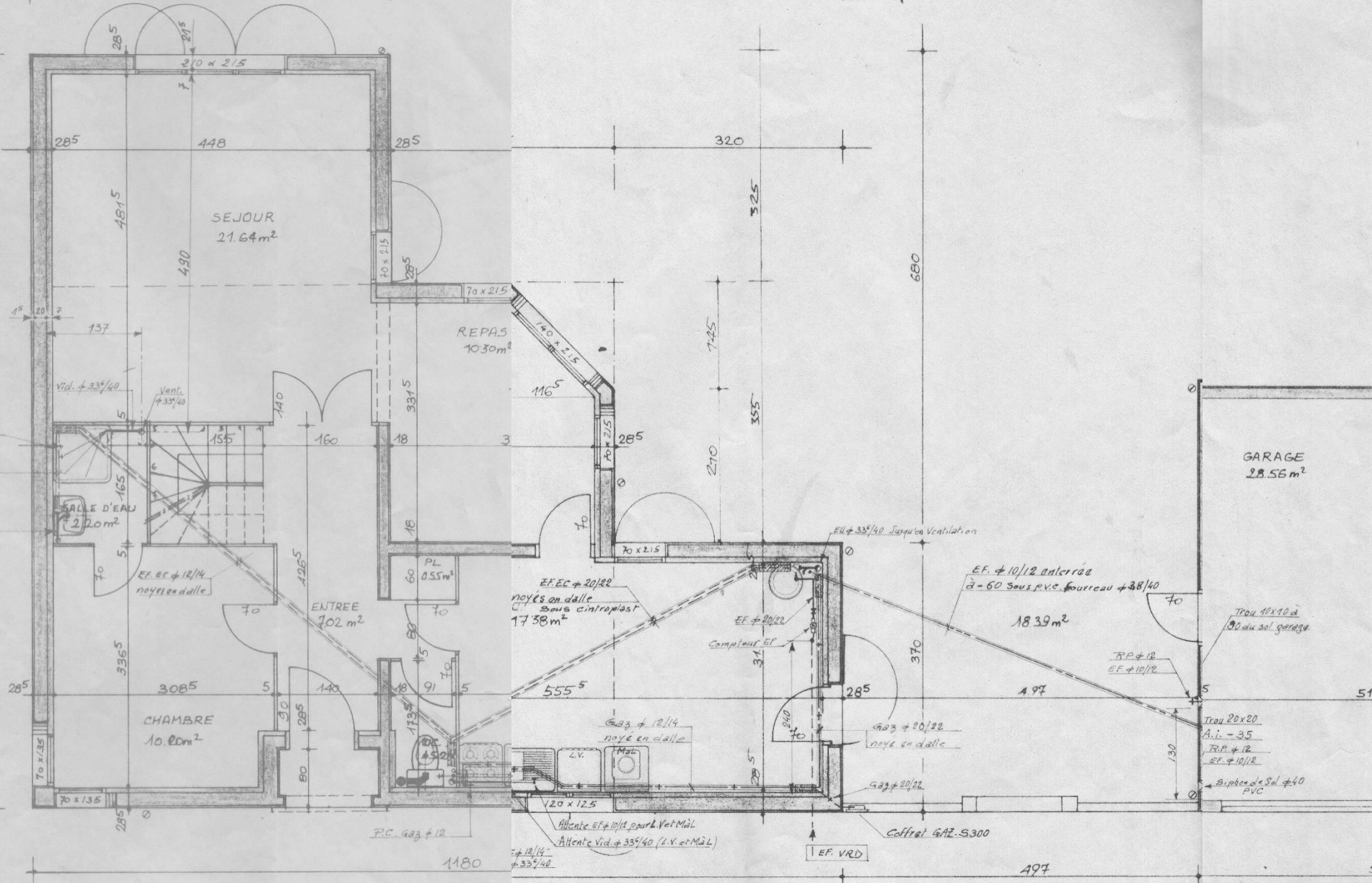
REZ DE CHAUSSEE 70.80m² Courtine (type C) : plan plomberie (original de 1980)
