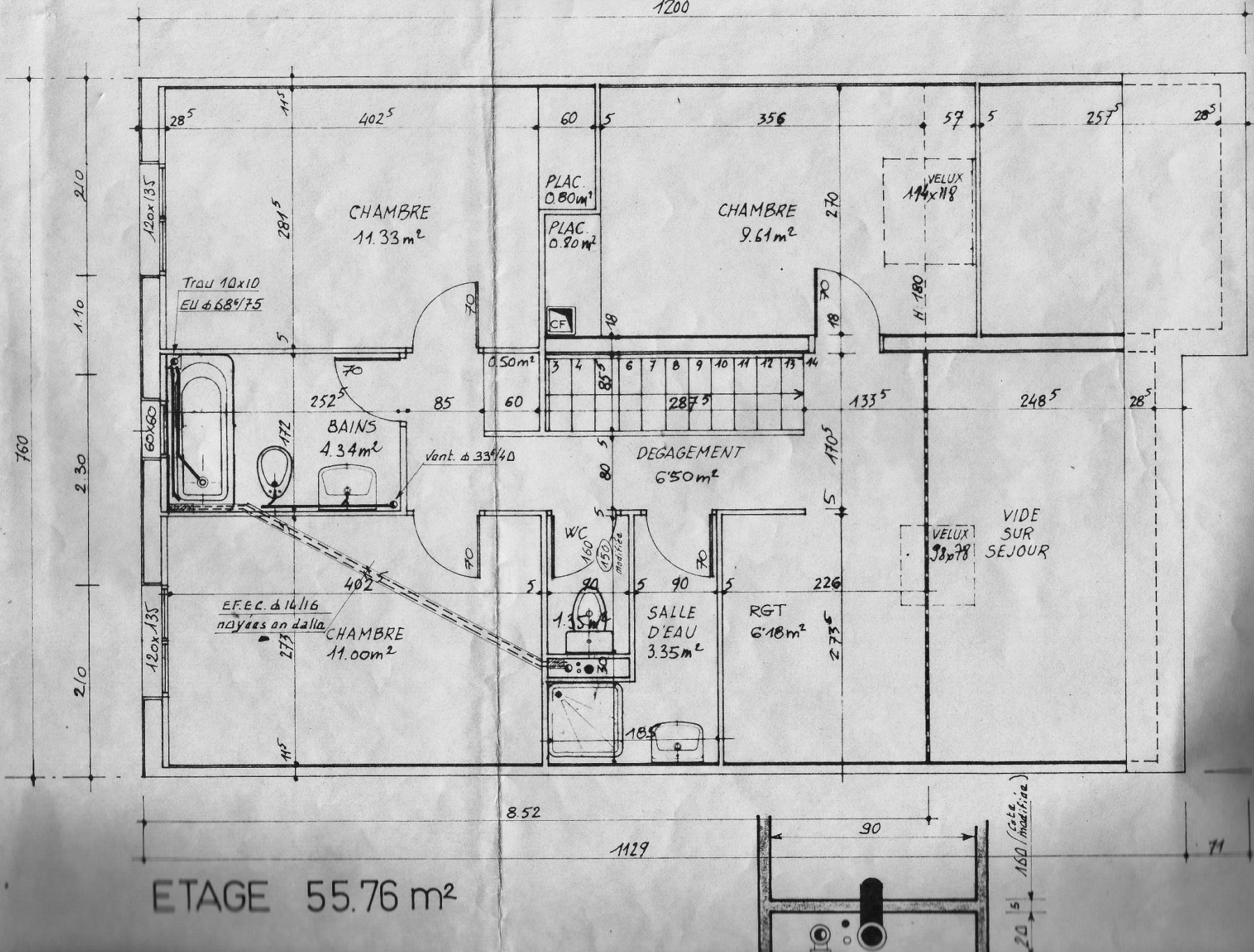
Bretèche (type B) : plan plomberie (original de 1980)
